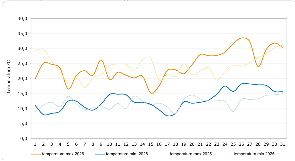
Grafico 1 – Temperature massime e minime. Maggio 2026 e 2025
