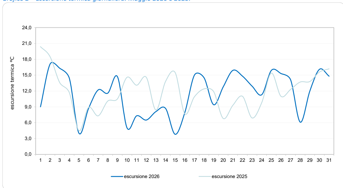
Grafico 2 – Escursione termica giornaliera. Maggio 2026 e 2025.
