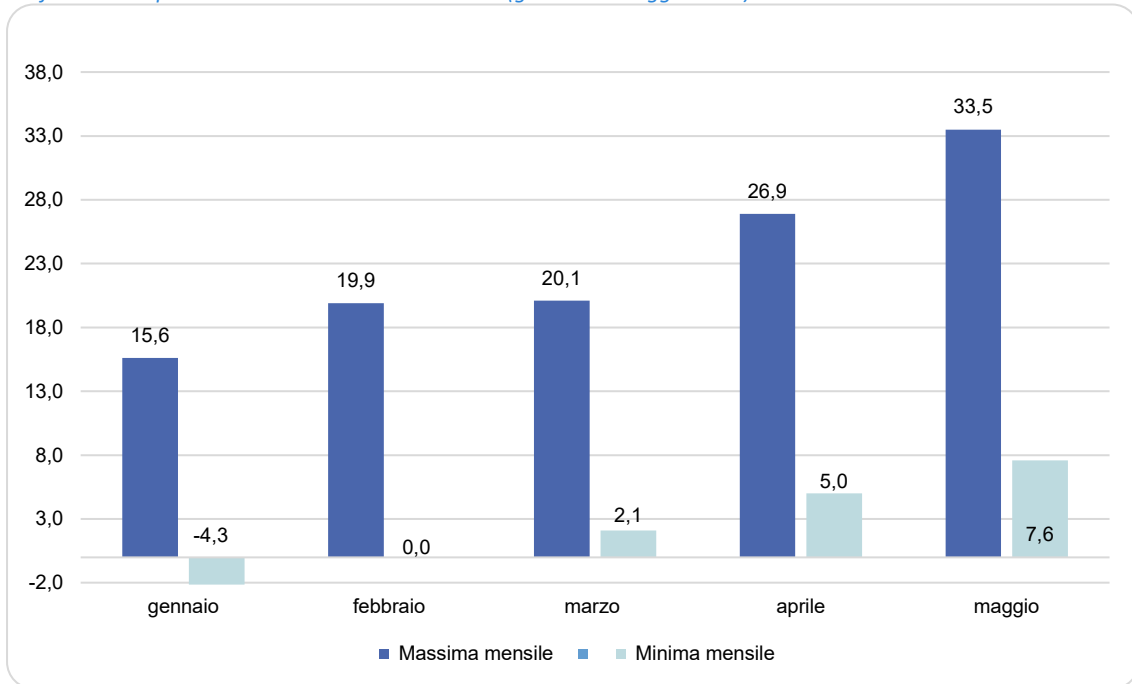
Grafico 3 – Temperature massime e minime mensili (gennaio – maggio 2026).
