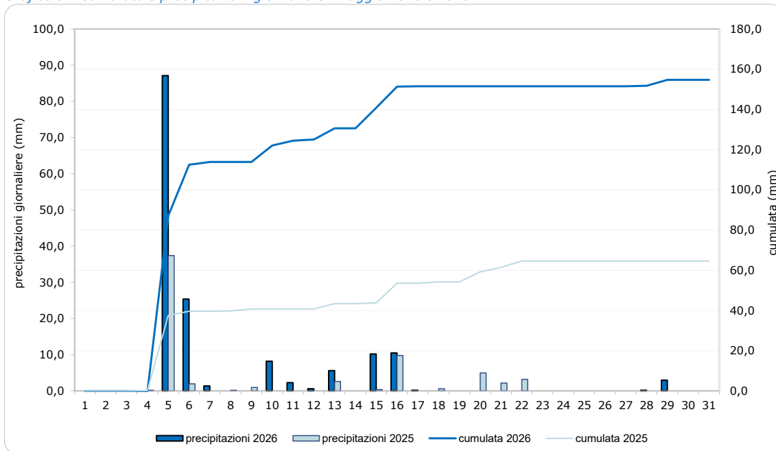
Grafico 5 – Cumulate e precipitazioni giornaliere. Maggio 2026 e 2025.
