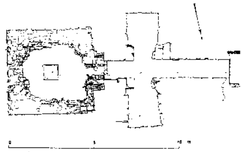
Fig. 3 - Vetulonia, Tomba della Pietrera, planimetria del livello superiore.
