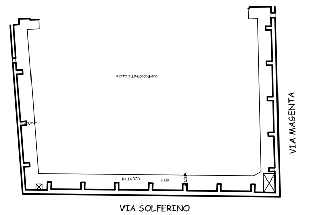
PIANO SESTO 2° ballatoio
