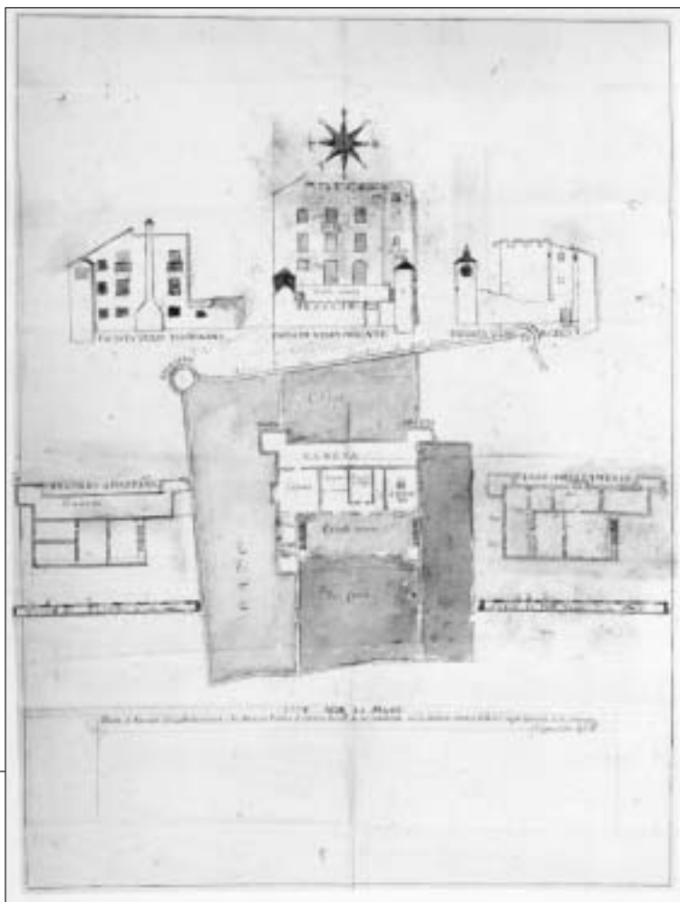
ORANO: pianta e prospetto del Castello di Orsera, sede estiva del vescovo parentino (autore: Riboni Lorenzo, agrimensore pubblico).
